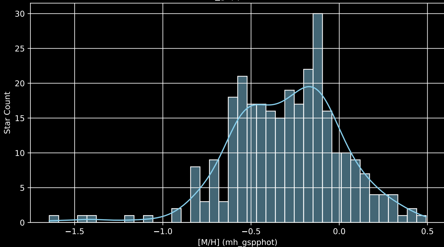
GALAH DR4 Field: [6861] [M/H] (mh_gspphot) (n= 290)
