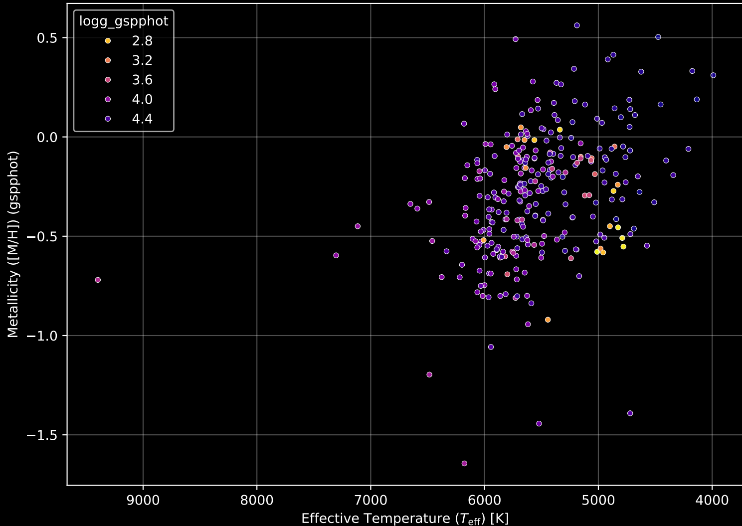
GALAH DR4 Field: [6861] Stellar Population Parameters (n= 292)
