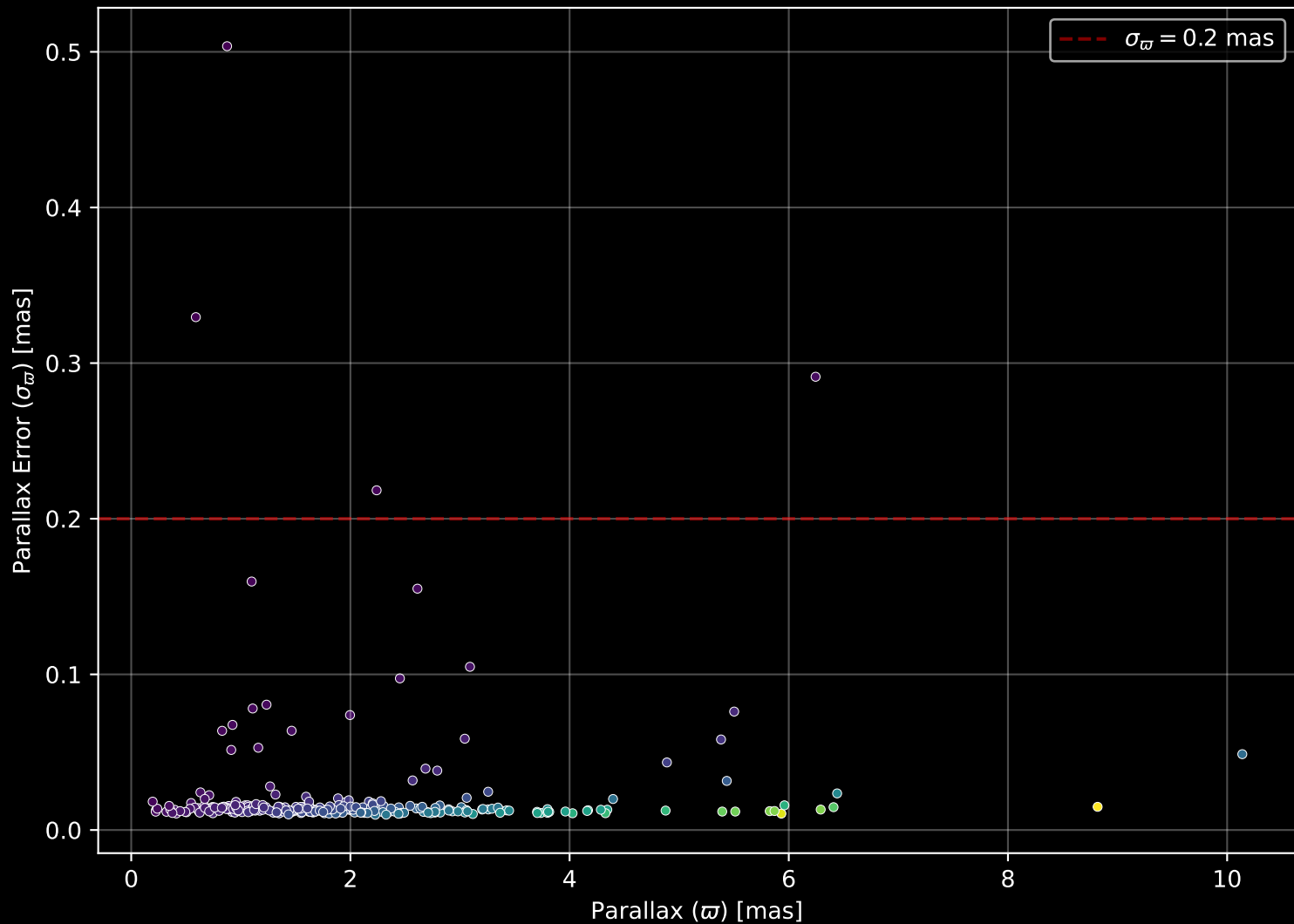
GALAH DR4 Field: [6861] Parallax Quality (n= 292)
